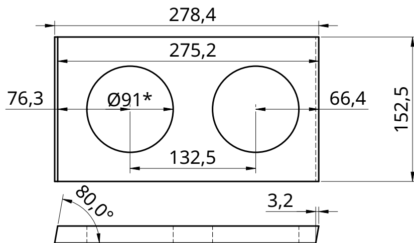
Planche 3 (dessin : planche gauche, vue de face)
